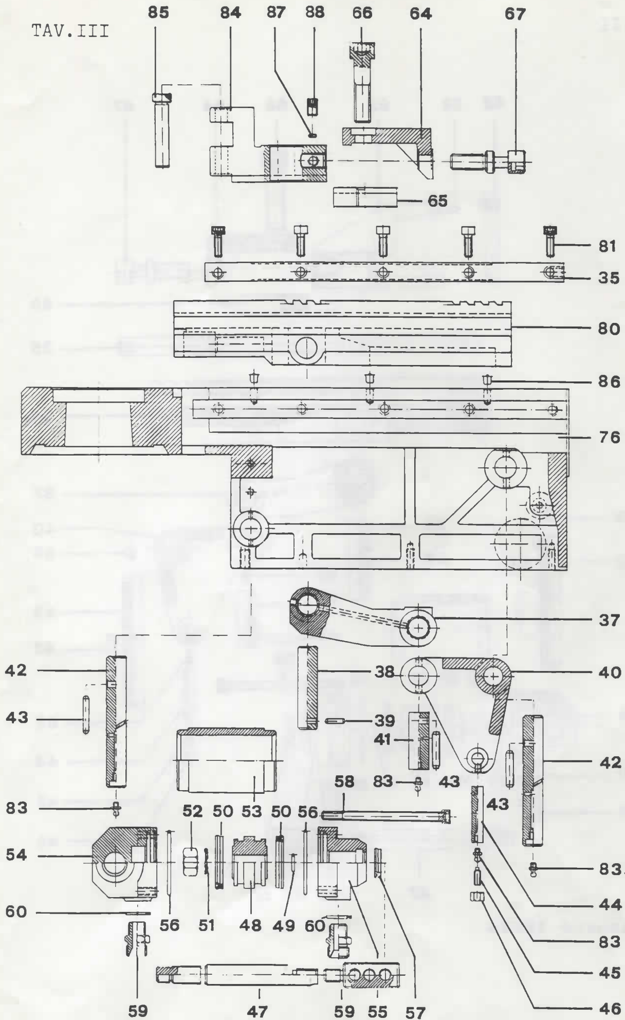
GRUPPO BRACCIO GIRAMATRICI
